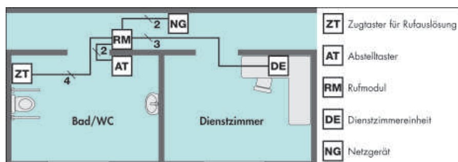
Anschlussschema
